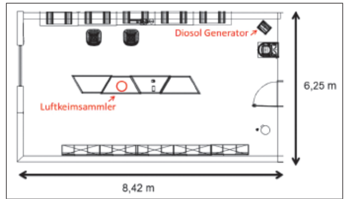
Abbildung 4: Schematischer Versuchsaufbau
