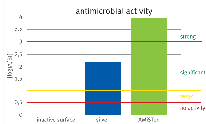
Abbildung 8: antimikrobielle Wirksamkeit der AMiSTec-Oberfläche im Vergleich zu einer Silberbeschichtung
