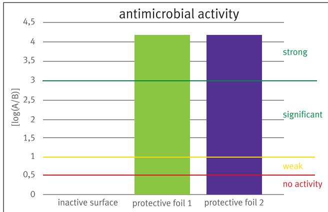
Abbildung 10: Antimikrobielle Wirksamkeit der getesteten Schutzfolien
