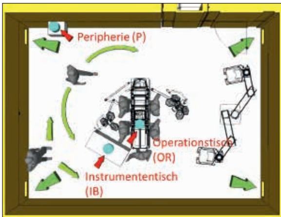
Abbildung 2: Messpunkte der Luftkeimmessungen (rote Pfeile) und Personenaktivität
