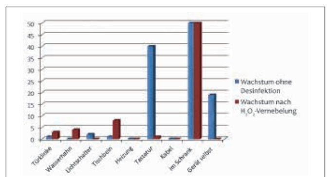
Abbildung 6: Keimzahlen (CFU) getesteter Oberflächen vor und nach Dekontamination
