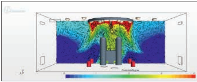
Abbildung 1: Schutzgradbestimmung im Forschungs-OP der OTH
